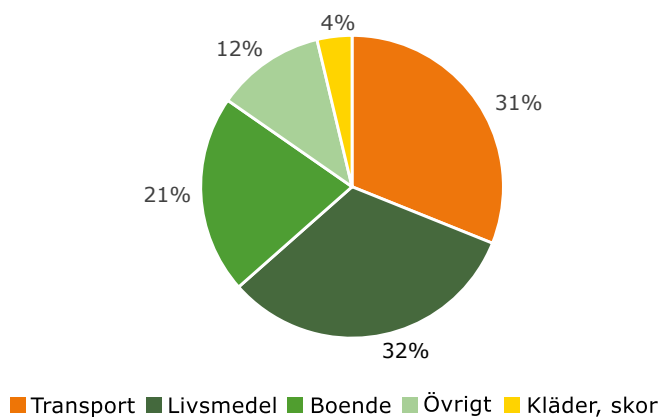
Konsumtionsbaserade utsläpp
